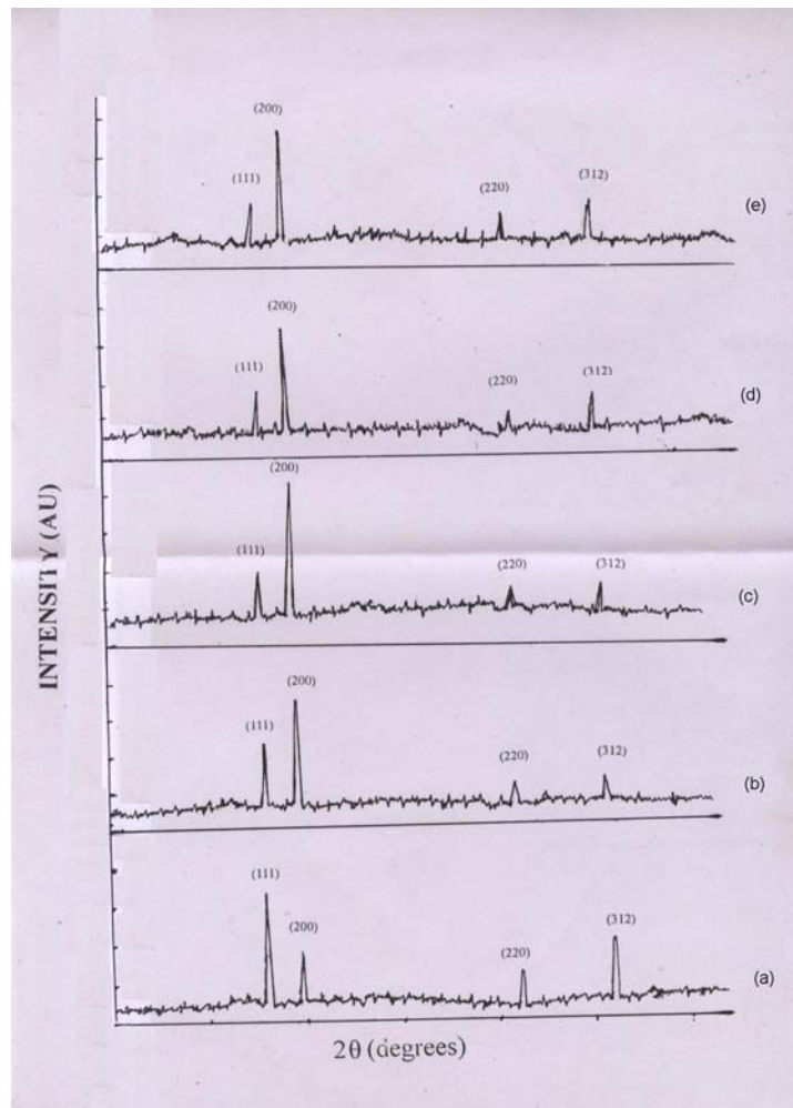
Fig. 3[(a), (b), (c), (d) & (e)] XRD patterns
